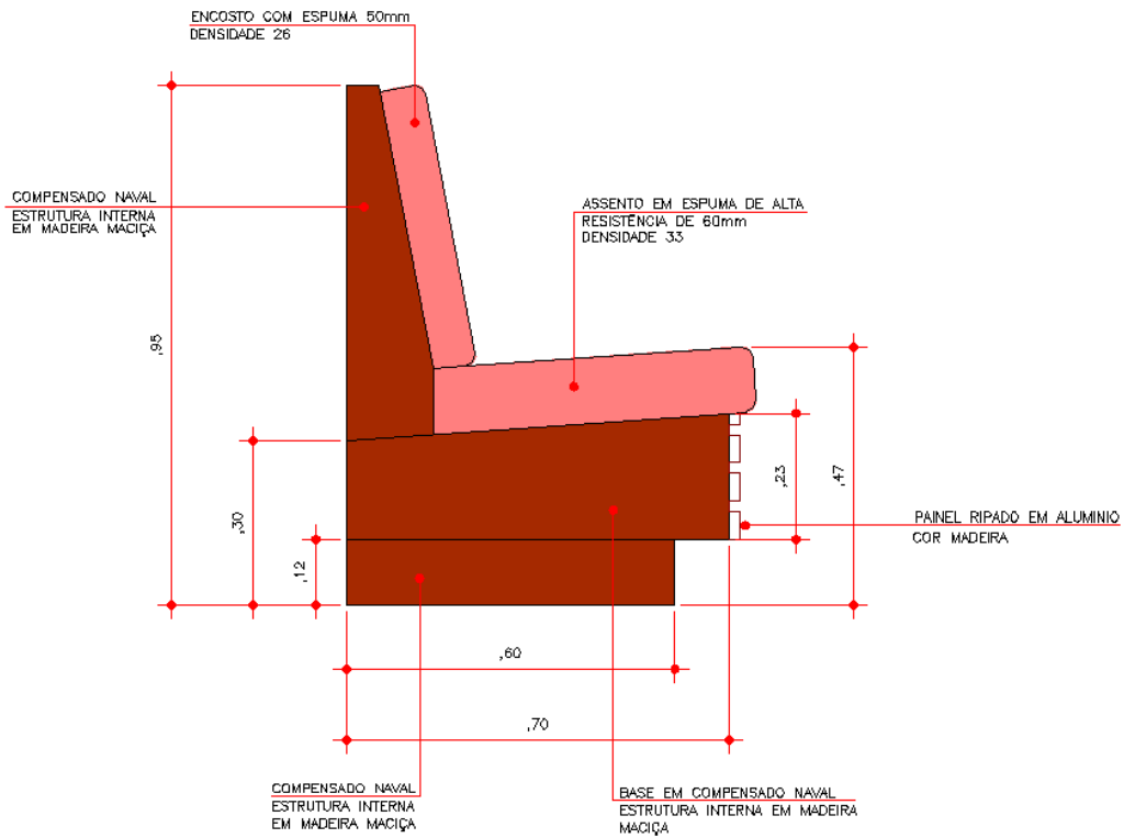
DETALHE 04 SOFÁ BOOTH ESTOFADO (MOD. CAPITONEE) VISTA LATERAL
